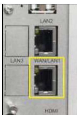
▲ N6850/N8850/N10850 Порт ГВС/ЛВС1
